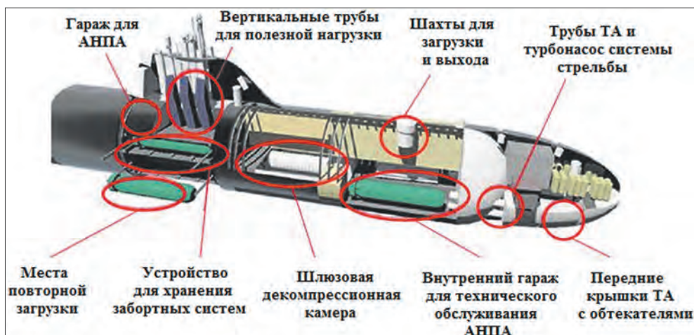
Один из вариантов компоновки ПЛА с размещением АНПА в районе миделя
