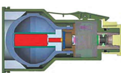
Светозумовой боеприпас ХМ809 комплекта (в разрезе)
