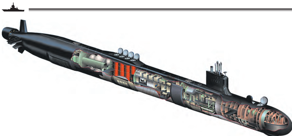
Многоцелевая ПЛА типа «Усовершенствованная Виргиния»
